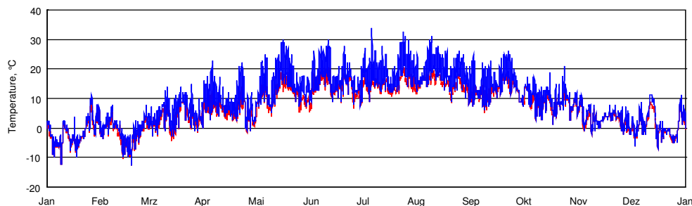
Fig.4 Temperaturverlauf in einem durchschnittlichen Jahr in Linz, blau Lufttemperatur, rot Feuchtkugeltemperatur.
