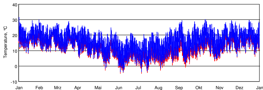
Fig.3 Temperaturverlauf in einem durchschnittlichen Jahr in Johannesburg, blau Lufttemperatur, rot Feuchtkugeltemperatur.
