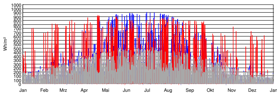
Fig.2 Solarstrahlung für Linz in Wh/m 2 : Blau Globalstrahlung; Rot Direktnormalstrahlung; Grau Diffusstrahlung
