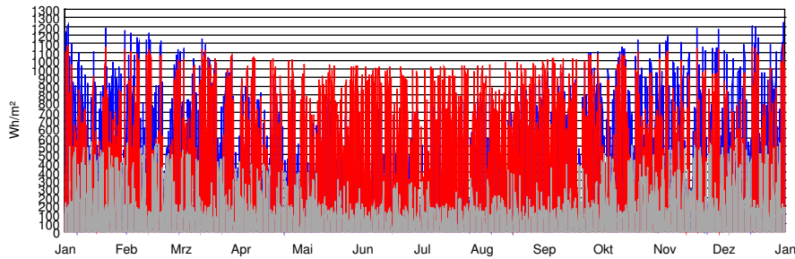
Fig.1 Solarstrahlung für Johannesburg in Wh/m 2 : Blau Globalstrahlung; Rot Direktnormalstrahlung; Grau Diffusstrahlung
